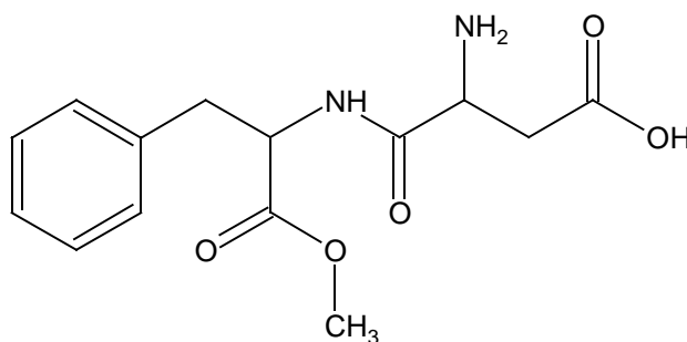
Aspartame
